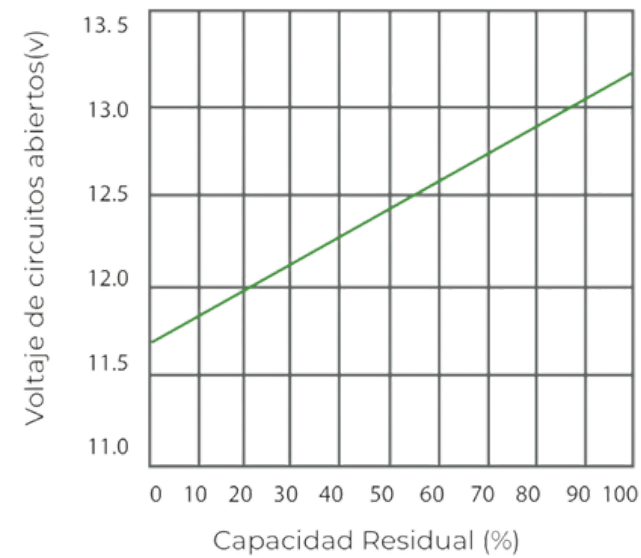
Voltaje en circuitos abiertos y capacidad residual
